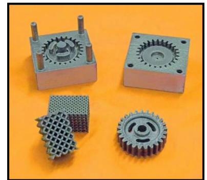
■開発鋼 Coフリーマルエージング鋼粉末による造形例
