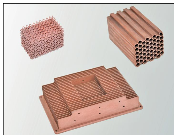
■ 開発鋼 3Dプリンター用銅合金粉末による造形例
