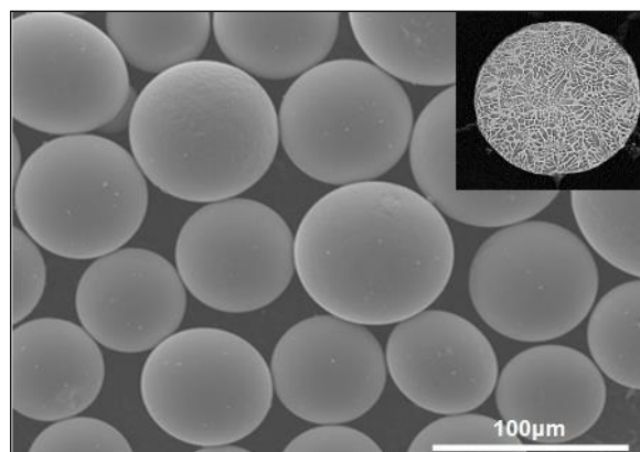
■ ガスアトマイズ粉末の電子顕微鏡写真およびマイクロ組織
