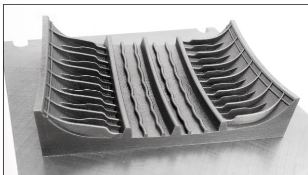
■ 3D積層造形 タイヤ成形金型(当社展示一例)
